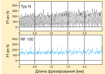
Сравнение сил резания между обычной фрезой типа N и фрезой RF 100 четко показывает более ровную, стабильную работу фрезы RF 100.
