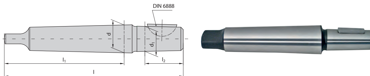
Хвостовик DIN 238 с полукруглой шпонкой DIN 6888 Arbor DIN 238 with woodruff key DIN 6888
